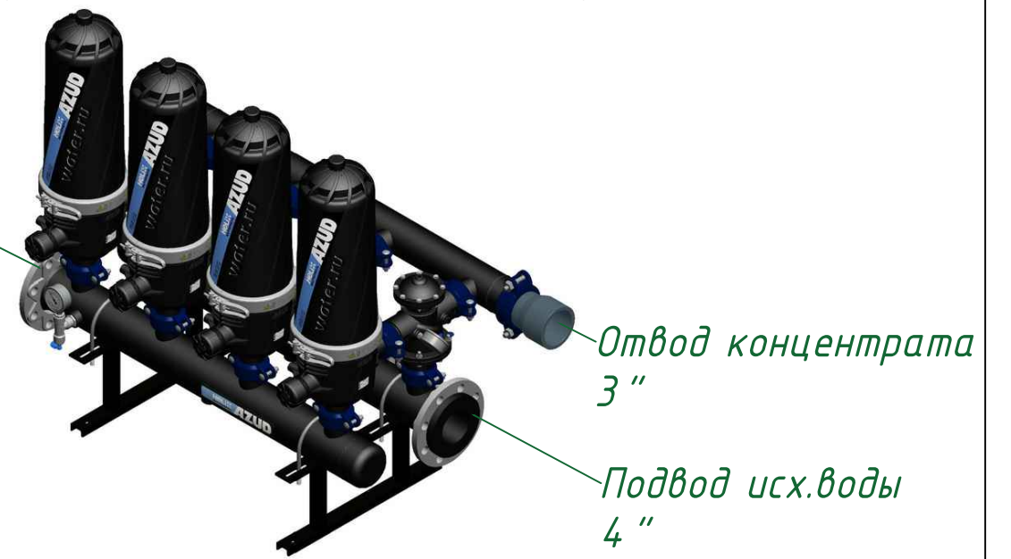
Изометрия
